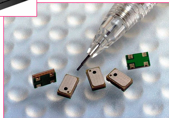
電子部品例
